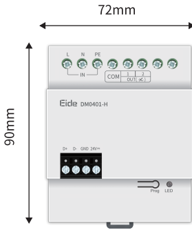
图2. 尺寸图—正面
