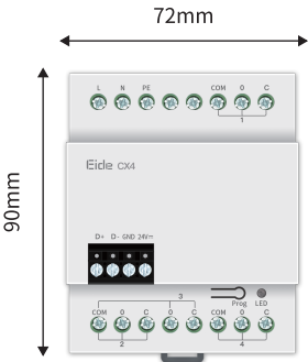
图2. 尺寸图—正面
