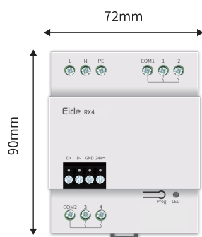
图2. 尺寸图—正面
